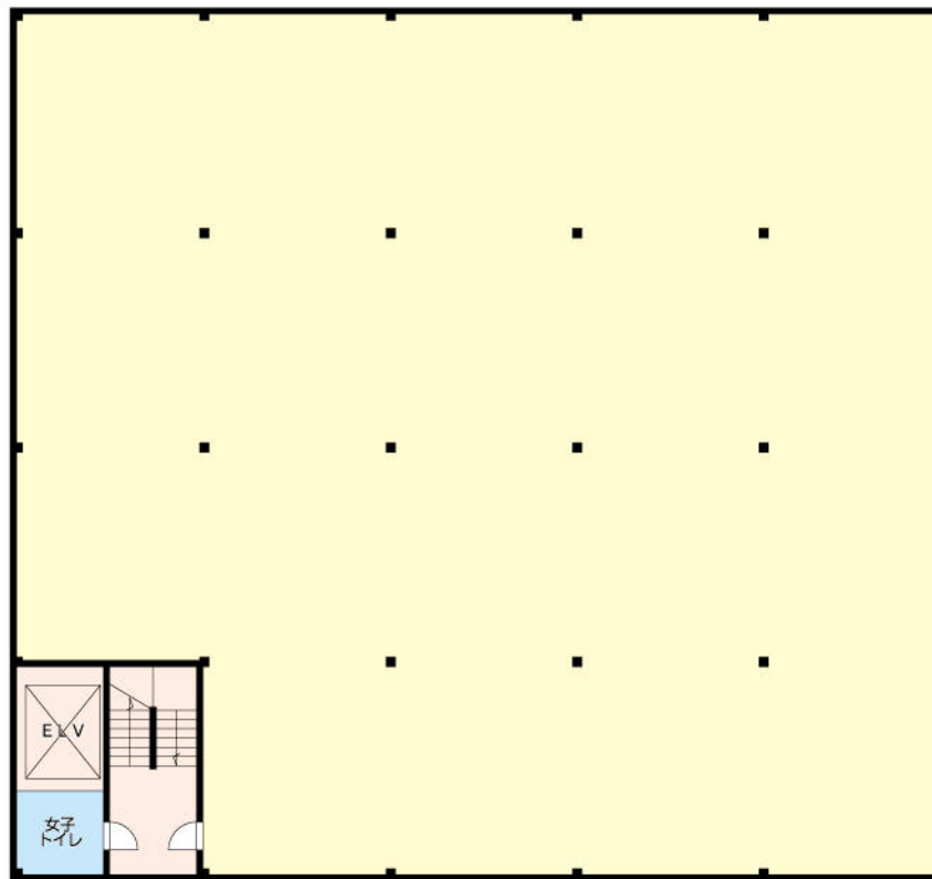
2階平面図
